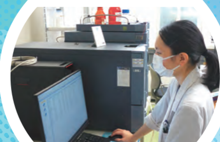
LC-MS/MS
